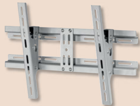
„Porta“ mit 15 Grad Neigung Art. Nr. 17765
